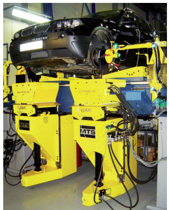
K&C: Ensayos de dinámica vehicular.
