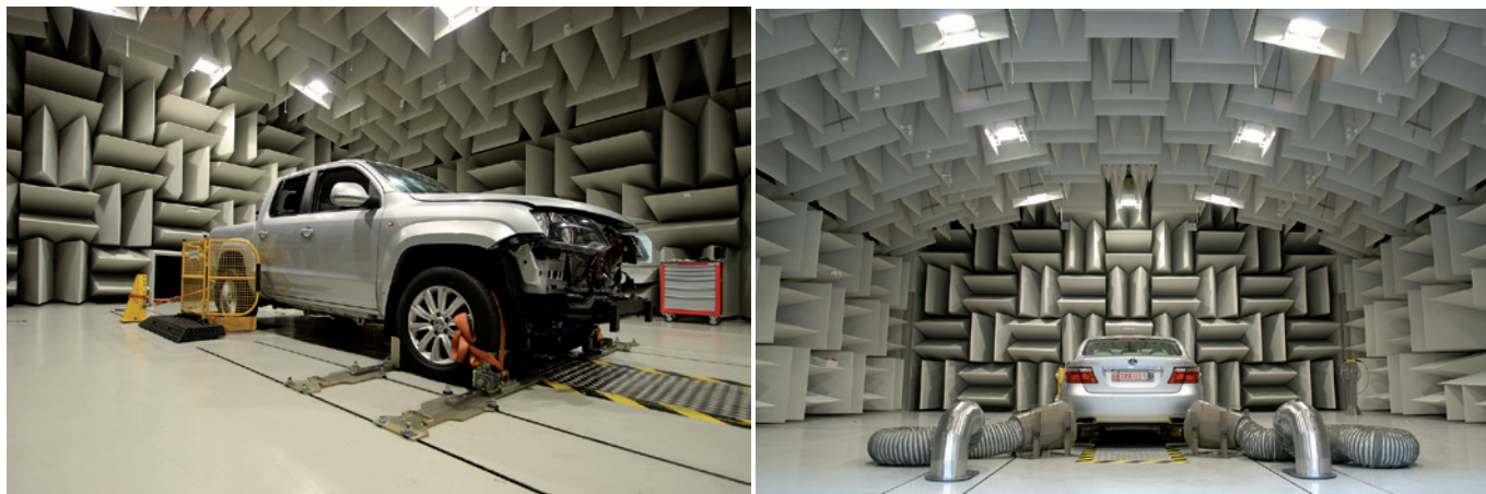
Cámara semi-anechoica.
